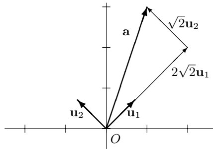
Abbildung 13.6. Orthogonalentwicklung: \mathbf{a} = 2\sqrt{2}\mathbf{u}_1 + \sqrt{2}\mathbf{u}_2
