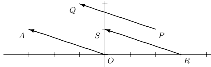
Abbildung 9.3. Verschiedenen Darstellungen des Vektors \mathbf{a} = (-3, 1)
