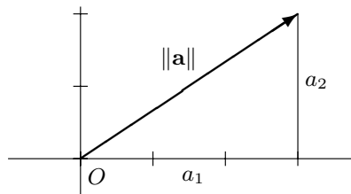
Abbildung 9.6. Länge eines Vektors
