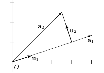
Abbildung 13.7. Gram-Schmidt-Verfahren
