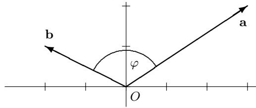
Abbildung 13.1. Winkel zwischen zwei Vektoren
