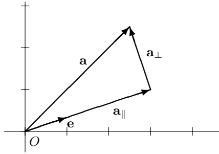
Abbildung 13.2. Orthogonale Projektion
