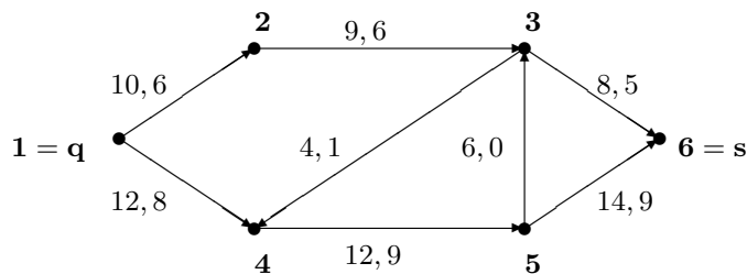
Abbildung 17.2. Durch das Netzwerk fließt ein Gesamtfluss 14.
