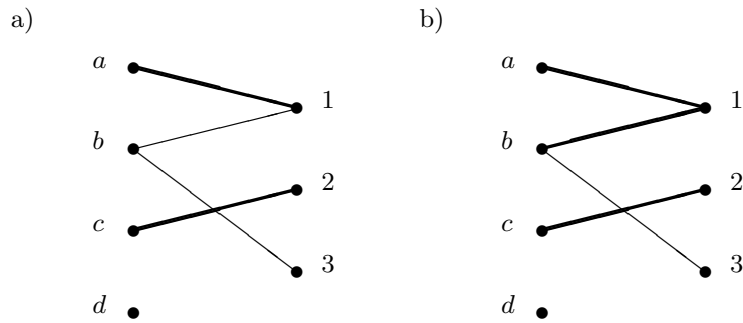
Abbildung 17.8. Handelt es sich um ein Matching?
