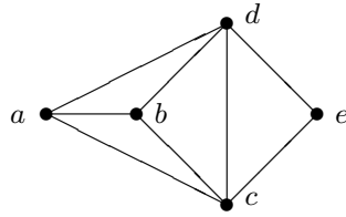
Abbildung 15.11. Kantenzug, Weg, Kreis
