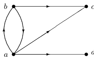
Abbildung 15.8. Digraph
