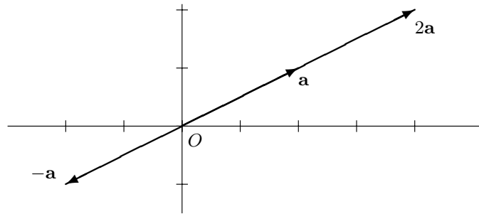
Abbildung 9.5. Multiplikation eines Vektors mit einem Skalar
