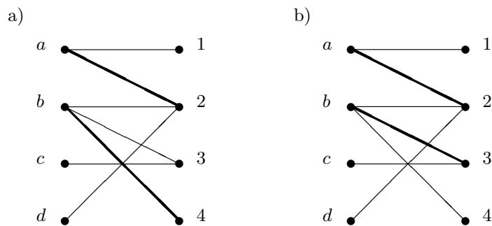
Abbildung 17.10. Alternierender Weg, Verbesserungsweg
