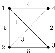
Abbildung 16.7. TSP: Gesucht ist eine billigste Rundreise.
