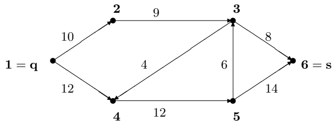
Abbildung 17.1. Netzwerk
