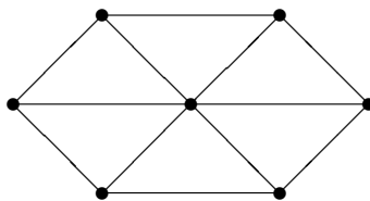
Abbildung 16.2. Kommunikationsnetz
