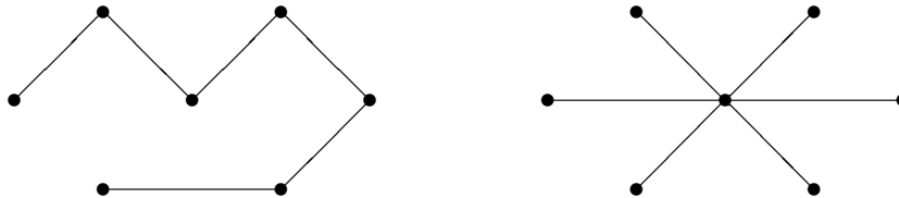
Abbildung 16.3. Aufspannende Bäume
