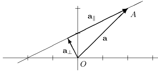
Abbildung 13.3. Abstand einer Geraden vom Ursprung
