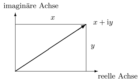
Abbildung 2.2. Gauß'sche Zahlenebene
