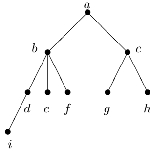
Abbildung 16.13. Baum zu Übungsaufgabe 16.6
