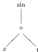
Abbildung 16.6. Der mathematische Ausdruck \sin(x+1) als Wurzelbaum
