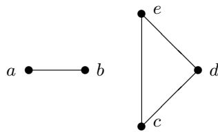
Abbildung 15.13. Nicht zusammenhängender Graph: Er besteht aus 2 Komponenten.
