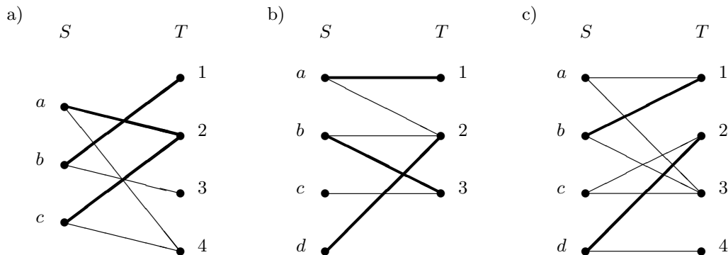
Abbildung 17.13. Matching?
