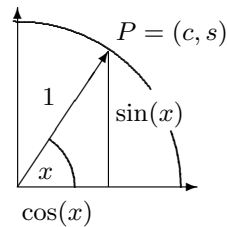
Abbildung 5.10. Definition von Sinus und Kosinus am Einheitskreis
