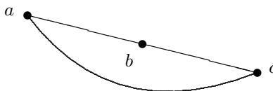
Abbildung 15.2. Teilgraph des Graphen aus Abbildung 15.1
