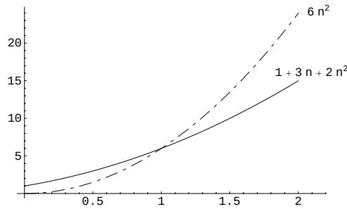
Abbildung 8.2. f(n) = 2n^2 + 3n + 1 und 6g(n) = 6n^2
