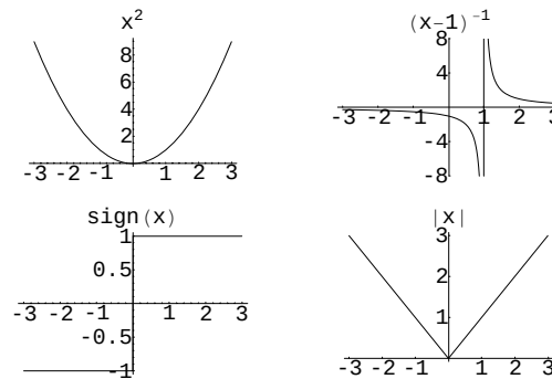
Abbildung 5.6. Die Funktionen aus Beispiel 5.25
