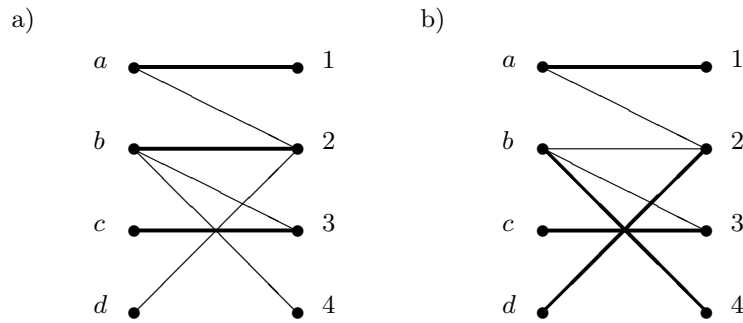
Abbildung 17.11. Konstruktion eines maximalen Matchings
