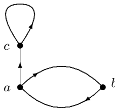
Abbildung 5.2. Relation auf der Menge A
