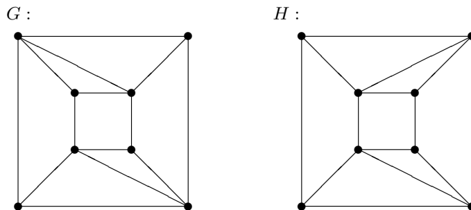
Abbildung 15.7. Sind diese Graphen äquivalent?
