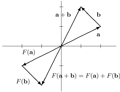
Abbildung 10.1. Spiegelung am Ursprung: F(\mathbf{a} + \mathbf{b}) = F(\mathbf{a}) + F(\mathbf{b})
