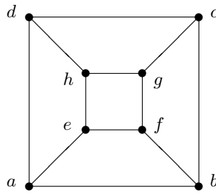
Abbildung 15.12. Kantenzug, Weg, Kreis
