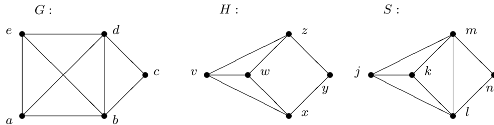
Abbildung 15.6. Sind die Graphen äquivalent?
