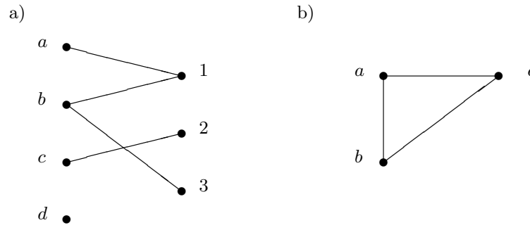
Abbildung 17.7. Bipartite Graphen?
