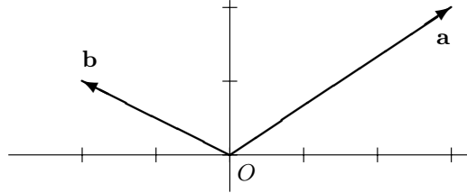
Abbildung 9.1. Darstellung eines Vektors im \mathbb{R}^2 als Ortsvektor
