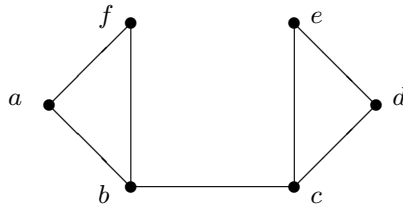
Abbildung 15.17. Adjazent, inzident, ...?
