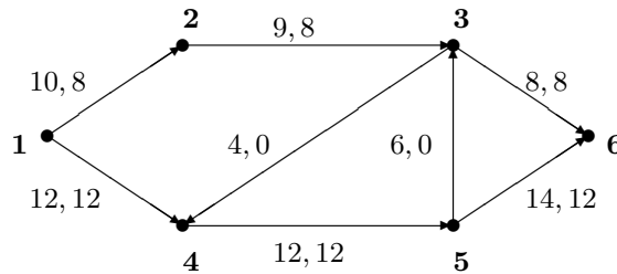
Abbildung 17.4. Maximaler Fluss
