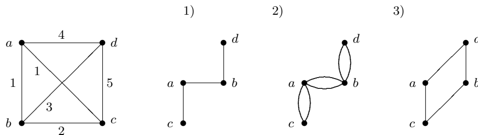
Abbildung 16.15. MST-Heuristik
