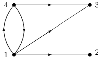
Abbildung 15.10. Digraph zu Beispiel 15.11
