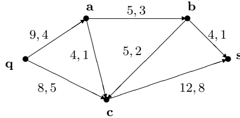
Abbildung 17.14. Wie groß ist der Gesamtfluss?
