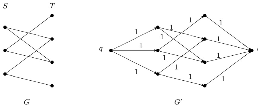
Abbildung 17.12. Bipartiter Graph G und zugehöriges Netzwerk G'
