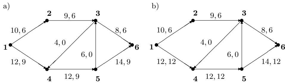
Abbildung 17.3. Vergrößerung des Flusses
