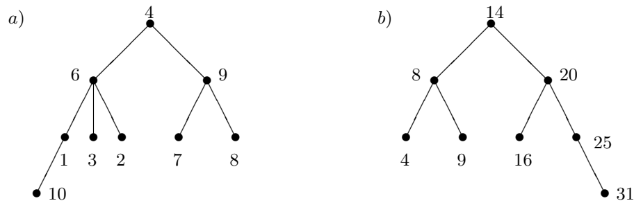
Abbildung 16.4. Wurzelbäume
