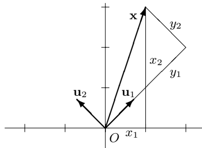
Abbildung 14.1. Basistransformation
