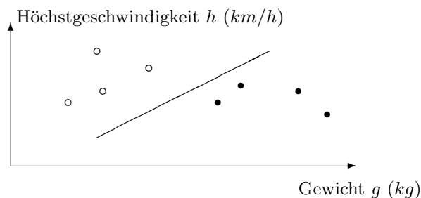
Abbildung 13.4. Lineare Klassifizierung
