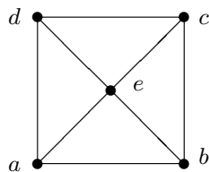
Abbildung 15.18. Graph zu Kontrollfrage 15.3.1
