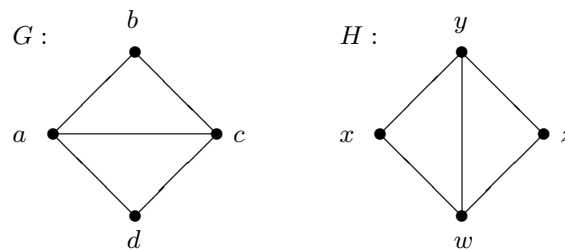
Abbildung 15.5. Graph G und Graph H sind äquivalent.
