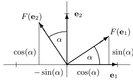
Abbildung 10.4. Drehung der Basisvektoren \mathbf{e}_1 und \mathbf{e}_2
