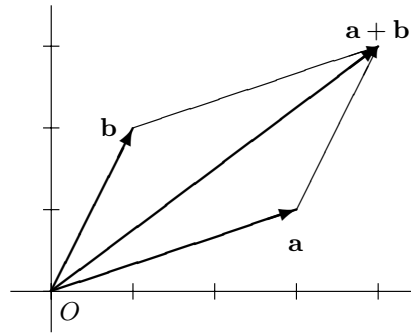
Abbildung 9.4. Addition zweier Vektoren
