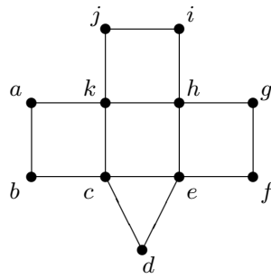
Abbildung 15.15. Euler-Zug oder das Problem des Schneepfluges
