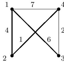
Abbildung 16.12. Ergebnis des Algorithmus von Dijkstra
