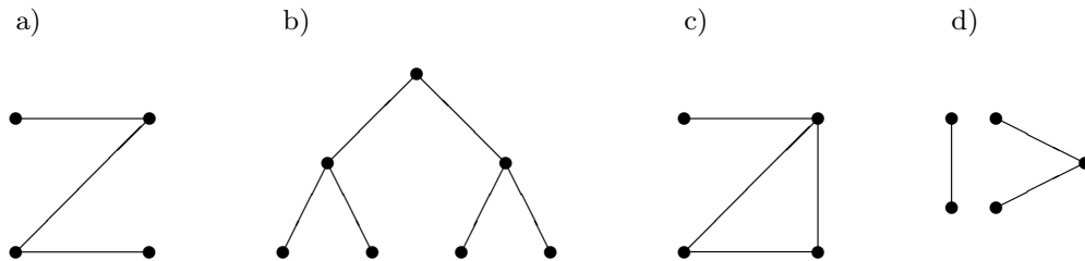
Abbildung 16.1. Handelt es sich um einen Baum?
