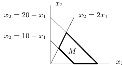
Abbildung 12.2. Der zulässige Bereich aus Beispiel 12.3.
