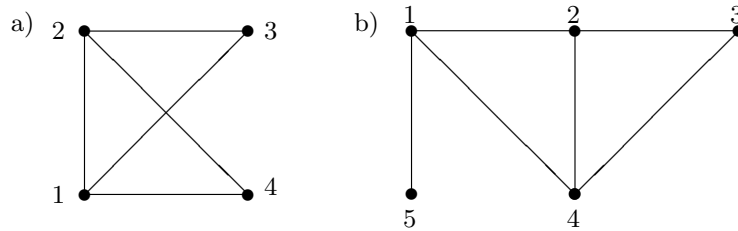
Abbildung 15.9. Die Graphen aus Beispiel 15.9
