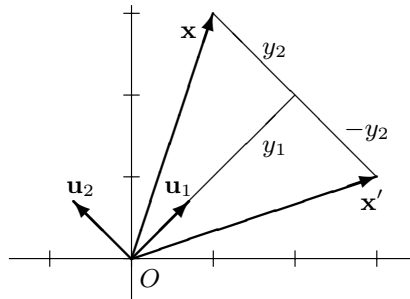
Abbildung 14.2. Spiegelung in verschiedenen Koordinaten
