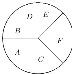
Abbildung 5.3. Äquivalenzklassen
