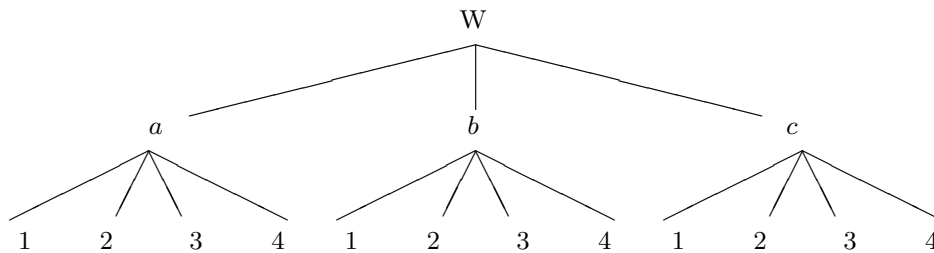
Abbildung 7.1. Baumdiagramm
