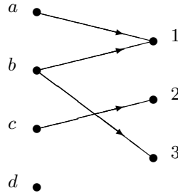
Abbildung 5.1. Graphische Darstellung einer Relation
