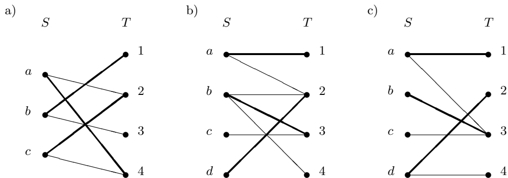
Abbildung 17.9. Handelt es sich um ein maximales Matching?
