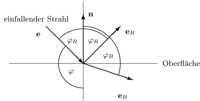
Abbildung 13.5. Brechung eines Lichtstrahls
