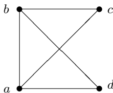
Abbildung 15.3. Eine Darstellung des Graphen aus Beispiel 15.2
