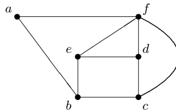
Abbildung 15.16. Hamilton-Kreis oder das Problem des Postboten
