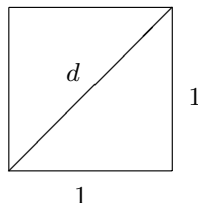
Abbildung 2.1. Quadrat mit Seitenlänge 1
