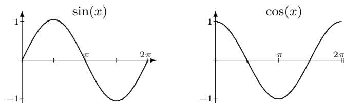
Abbildung 5.11. Sinus- und Kosinusfunktion
