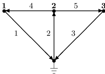
Abbildung 10.5. Elektrisches Netzwerk
